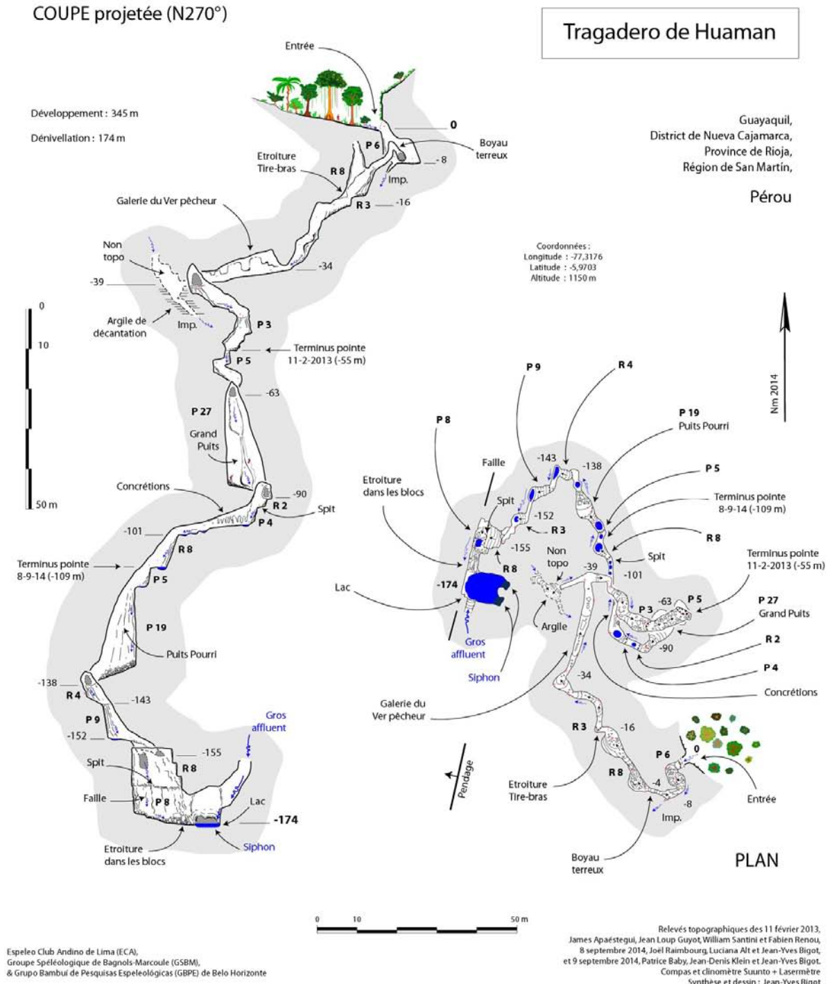
Fig. 6 : Topographie du tragadero de Huaman.
