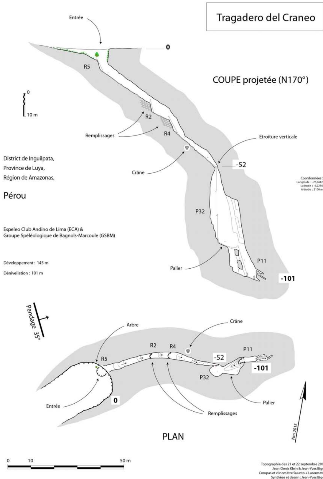
Fig. 5 : Topographie du Tragadero del Craneo.
