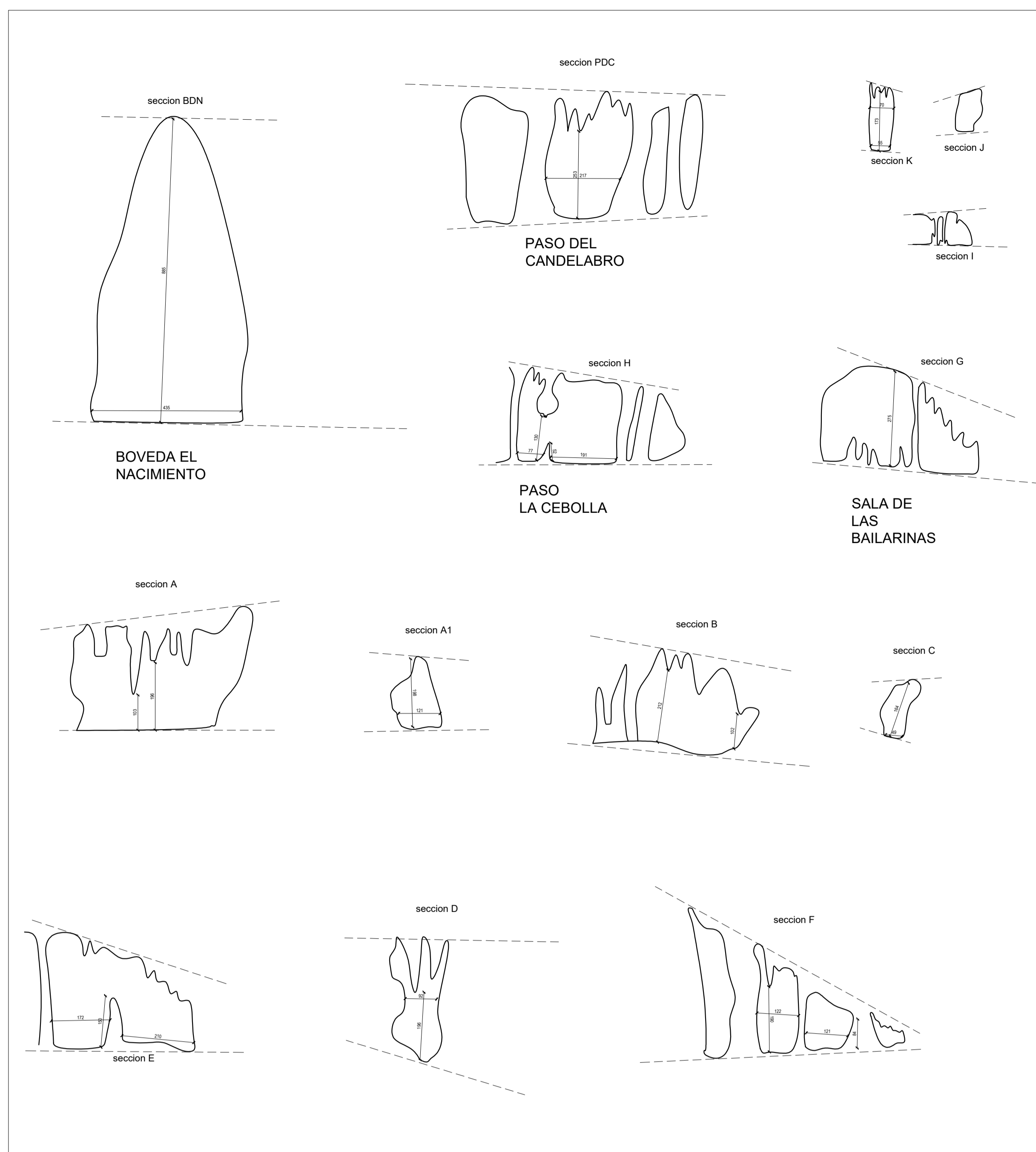
SECCIONES TRANSVERSALES
