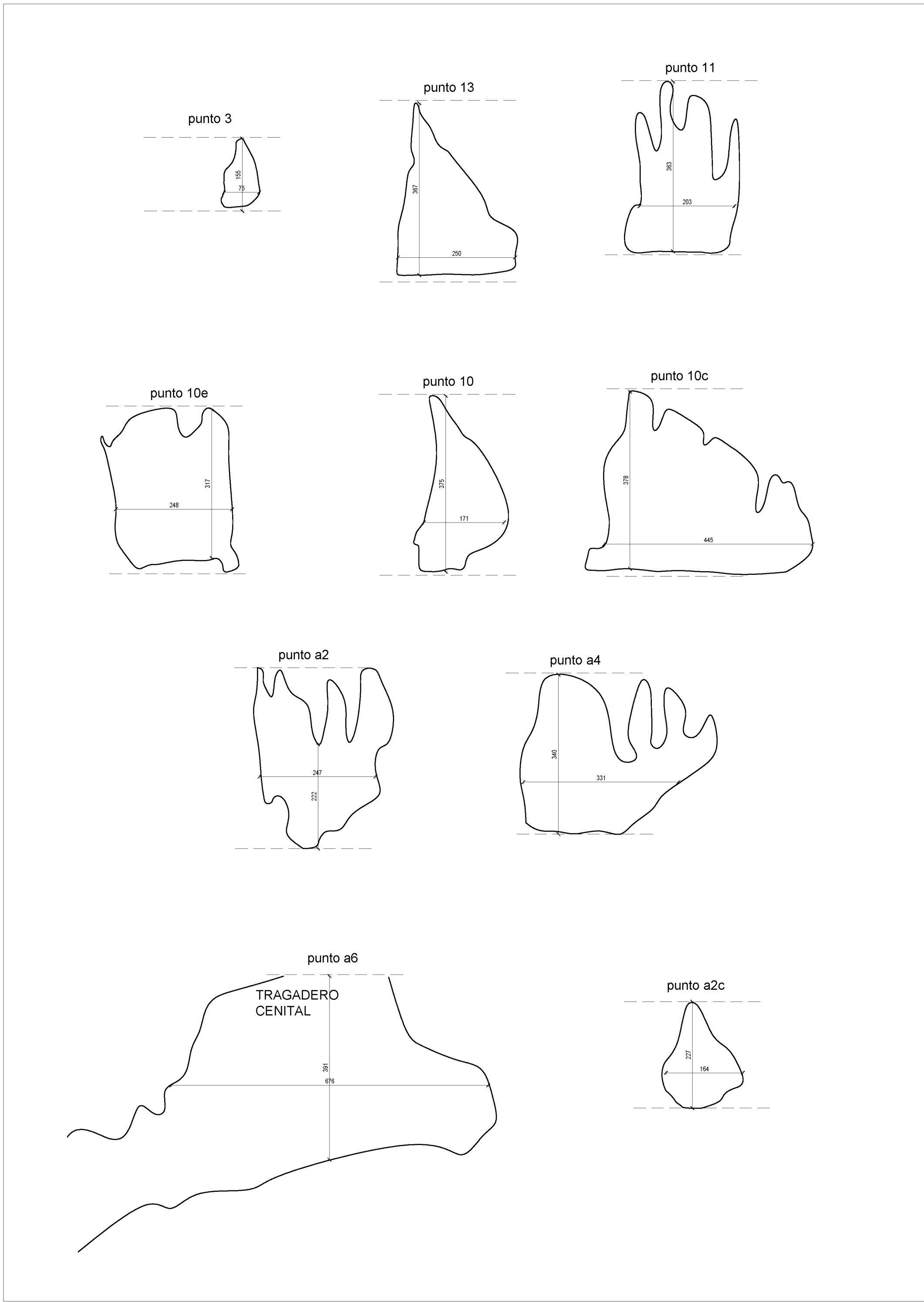
SECCIONES TRANSVERSALES
