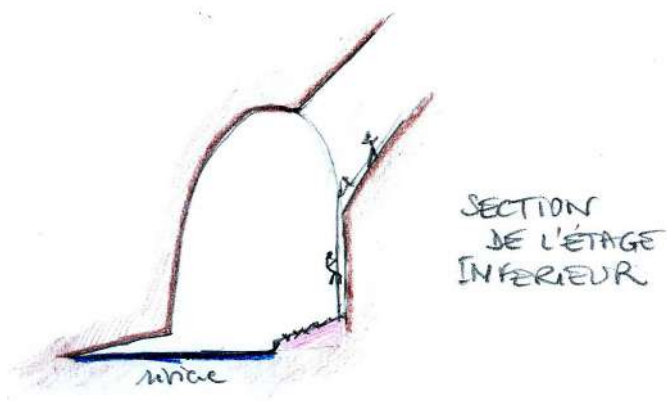
Fig. 5 : Section de la rivière souterraine comportant une encoche latérale marquée.
