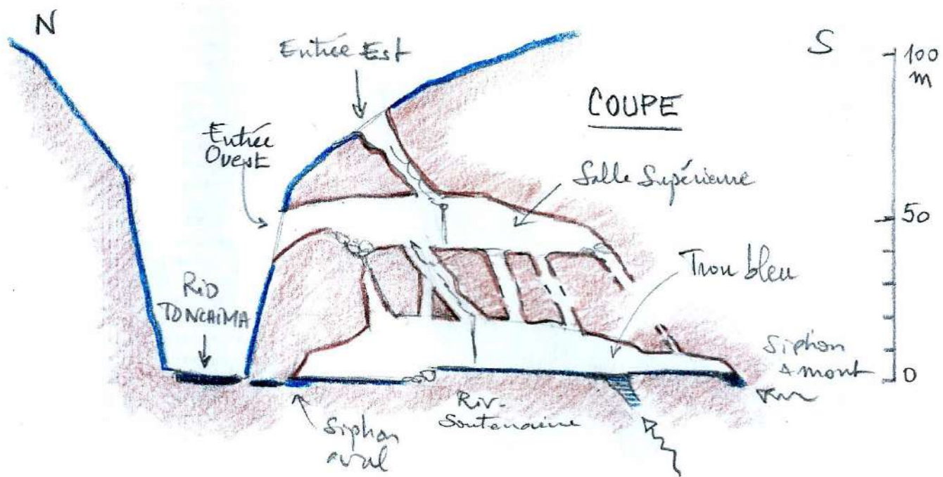
Fig. 2 : Coupe schématique représentant l'étagement des galeries.
