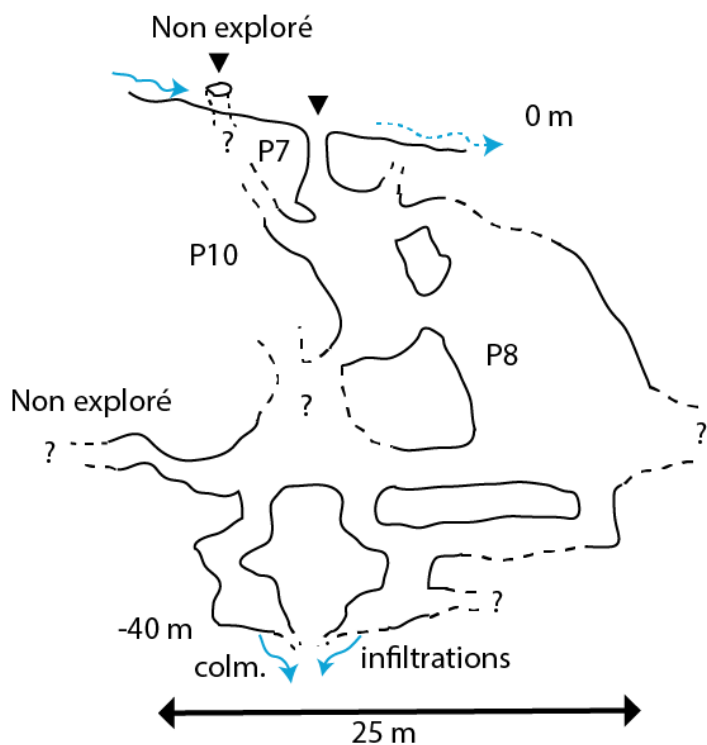
Coupe schématique 2017 : Mathias Echevin
