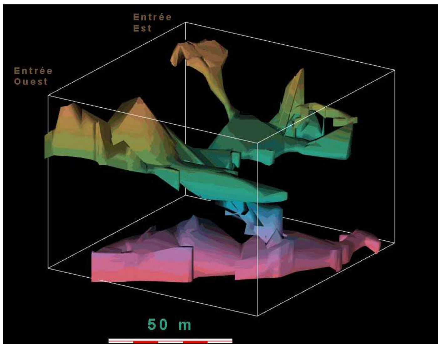
Fig. 3 : Vue 3D de la Cueva de los Guacharos de Soritor. On distingue deux niveaux de creusement matérialisés par les galeries horizontales. Extrait du logiciel Therion, Xavier Robert, 2017.
