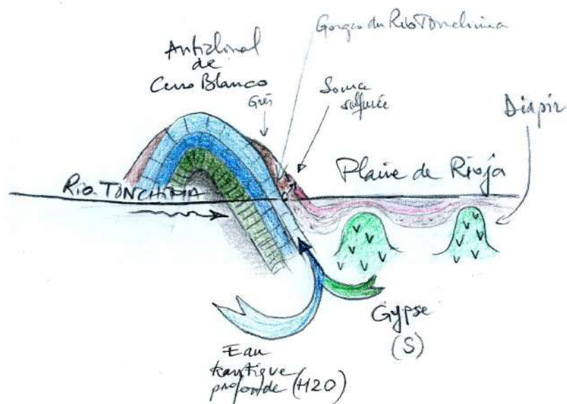
Fig. 7 : Coupe géologique simplifiée de l'anticlinal de Cerro Blanco et de la plaine de Rioja. Les caractéristiques des eaux seraient liées à la présence de gypse.
